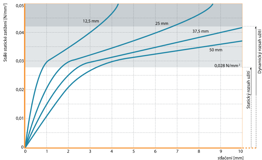
Obr. 1: Křivka stlačení při kvazistálém zatížení, měřeno se zatěžovací rychlostí 0,0028 \text{ N/mm}^2/\text{s}
