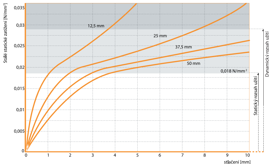
Obr. 1: Křivka stlačení při kvazistálém zatížení, měřeno se zatěžovací rychlostí 0,0018 \text{ N/mm}^2/\text{s}
